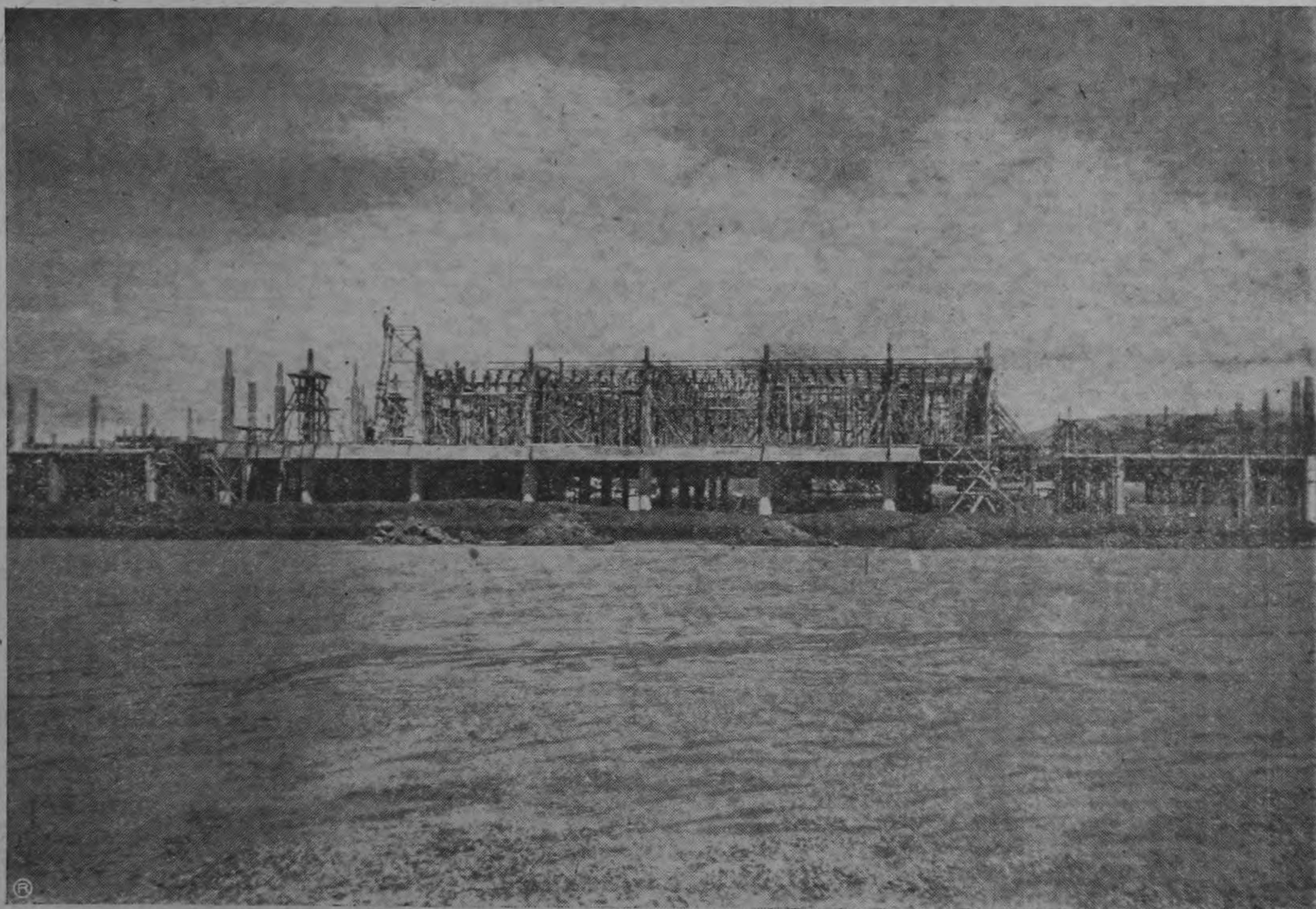
LAS INSTALACIONES DE EL COCO. — Rápidamente avanzan los trabajos del aeropuerto de El Coco. La vista da idea cabal de la magnitud de las obras. Del edificio central, planeado para cuatro pisos, ya están levantadas las estructuras de dos. En primer plano, la vasta pista de estacionamiento de aviones, cuyo lastrado está prácticamente listo: falta sólo la capa de concreto. (Foto Arévalo)
